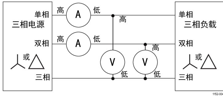
图 27: 三相三线 (双功率表法)。选择三相三线
