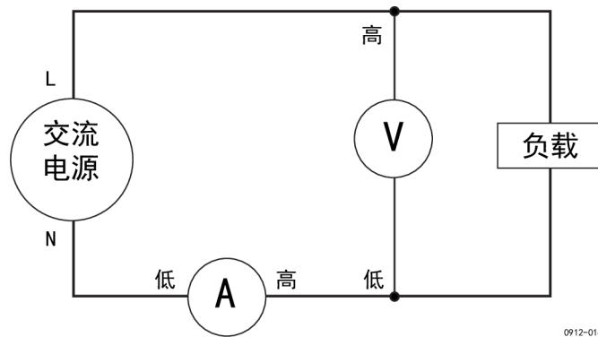
图 1: 典型的 PA3000 输入连接
