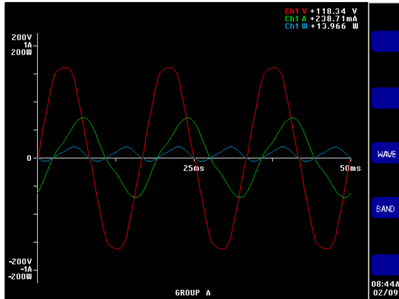
图 8: 波形屏幕
