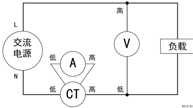
图 18: 变流器连接
