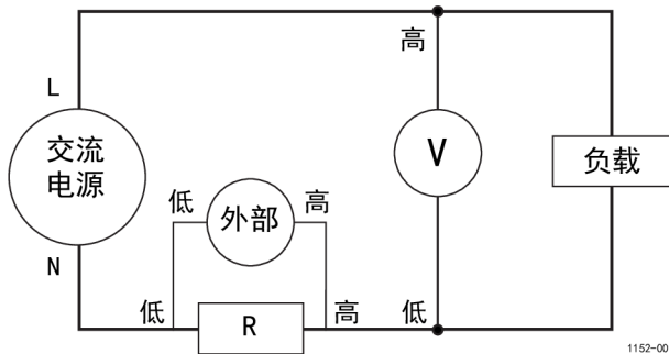
图 21: 外部电阻分流器连接
