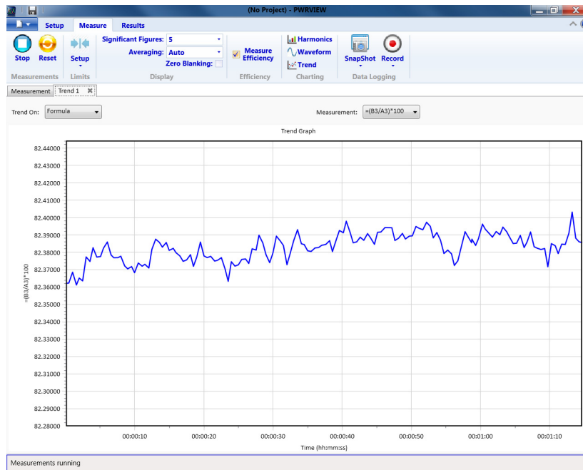
图 42: 效率趋势图
