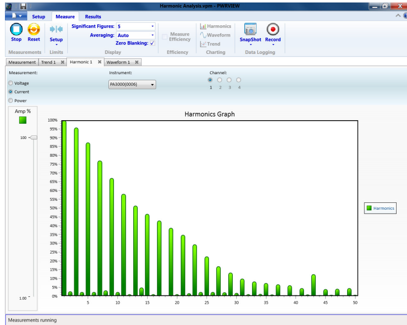
图 49: 谐波条形图
