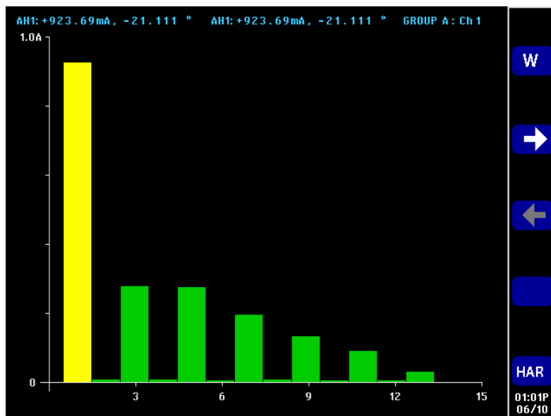
图 9: 条形图屏幕
