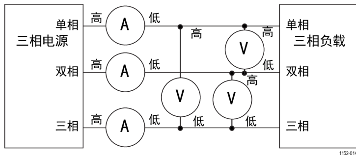
图 28: 三相三线 (三功率表法)。选择三相三线 (3V3A)。
