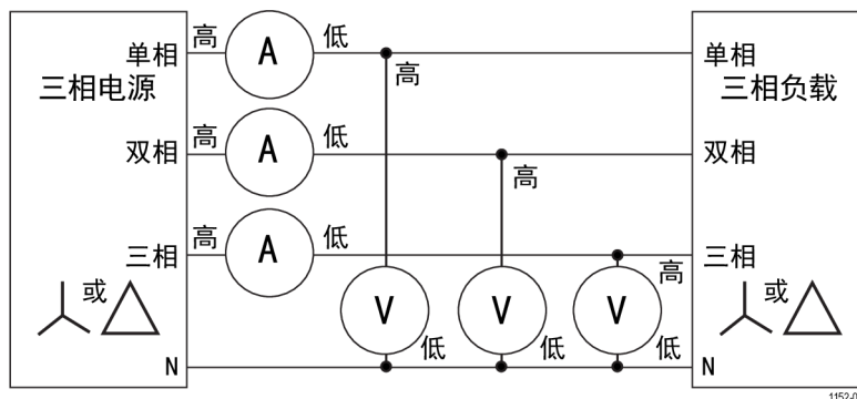
图 30: 三相四线 (三功率表法)。选择三相四线
