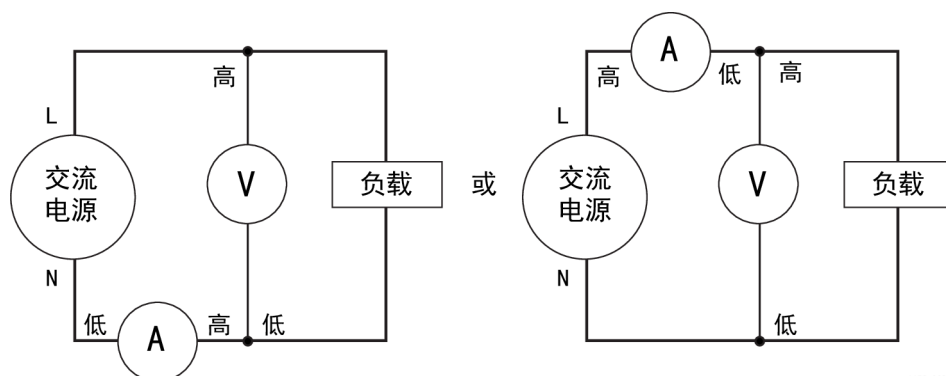
图 25: 单相两线和直流测量。选择单相两线模式
