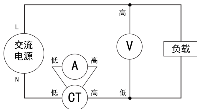
图 20: 变流器连接
