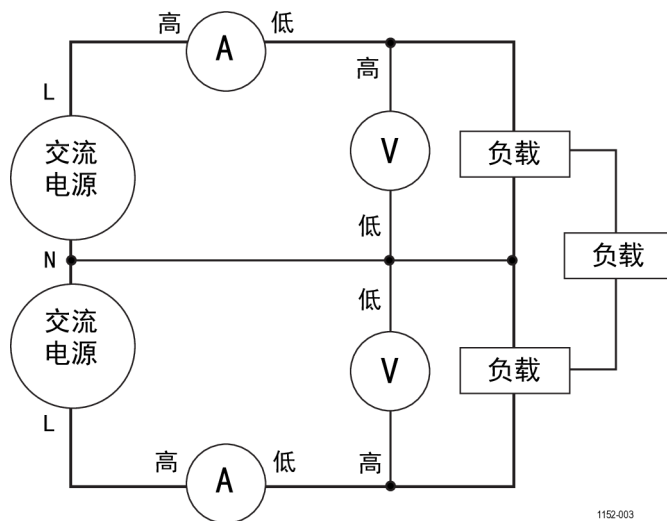
图 26: 单相三线。选择单相三线
