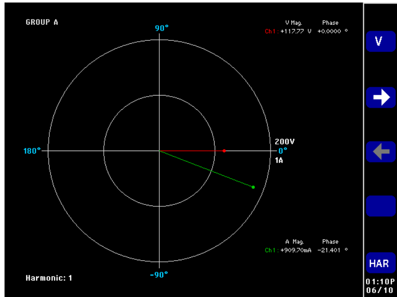
图 11: 矢量图屏幕
