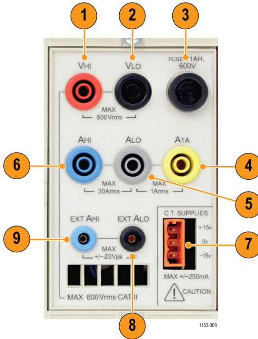
图 17: 后面板上的信号输入 (显示通道 1)
