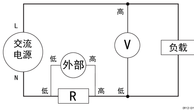
图 19: 外部电阻分流器连接
