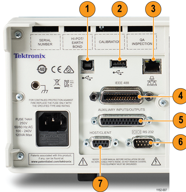
图 61: 后面板上的功率分析仪通信端口
