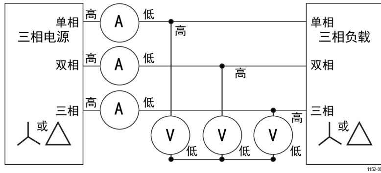
图 29: 三相三线 (三功率表法)。选择三相四线
